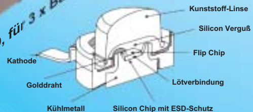
Collimator Linsenaufbau
